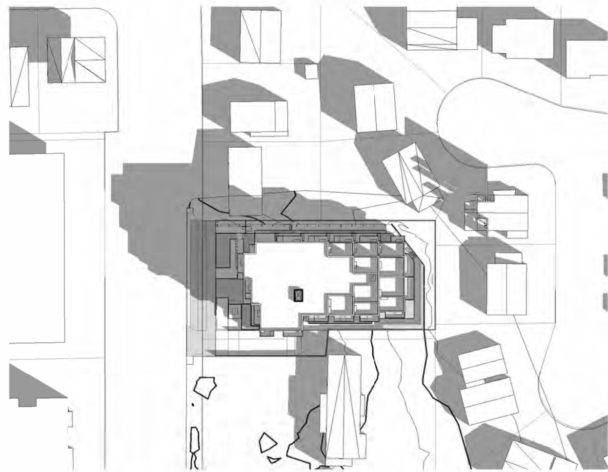
1 Spring/Fall Equinox - 03/20 9am DP.403 1 : 1000
