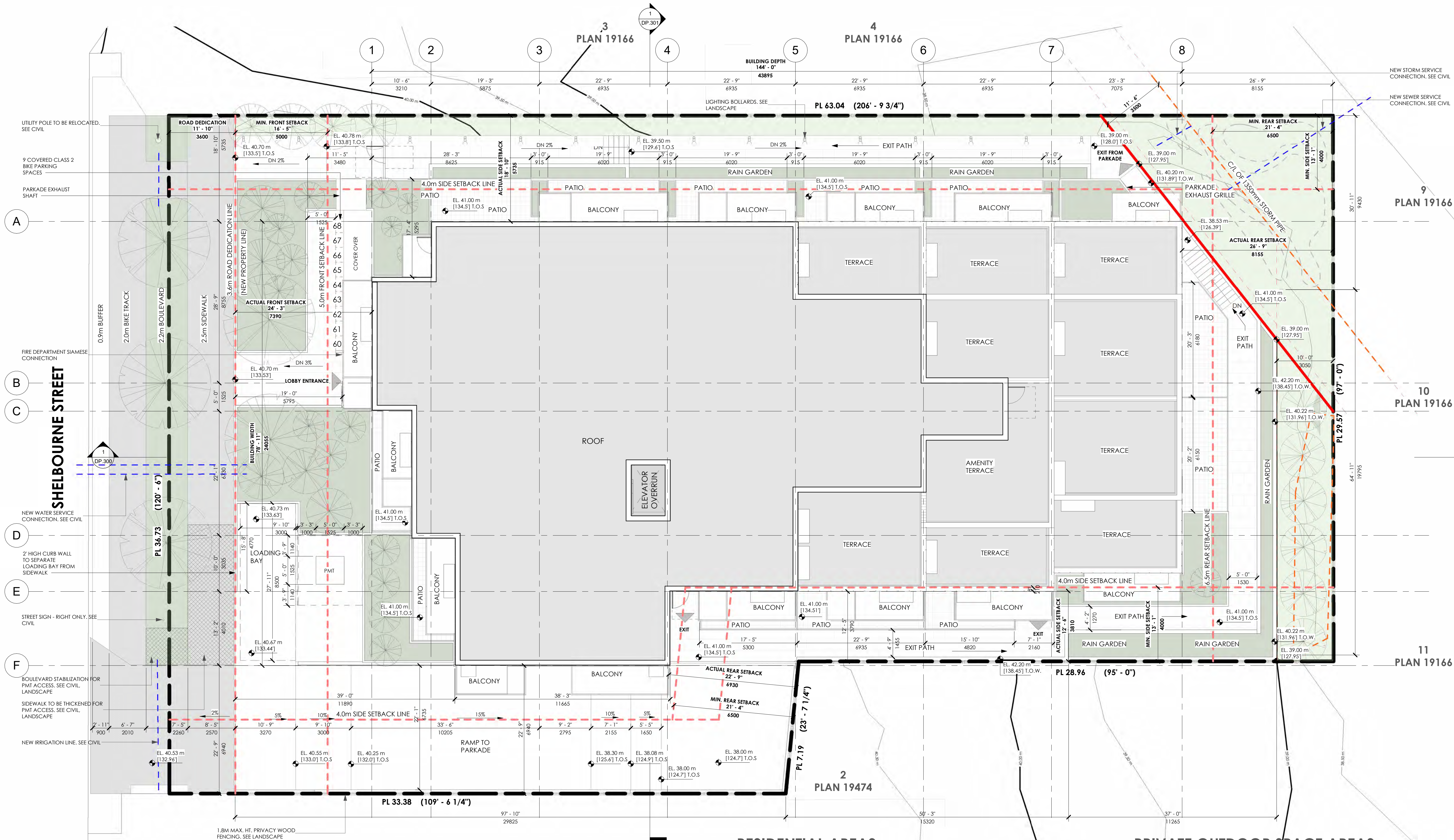
1 SITE PLAN - DP DP.100 1 : 100
